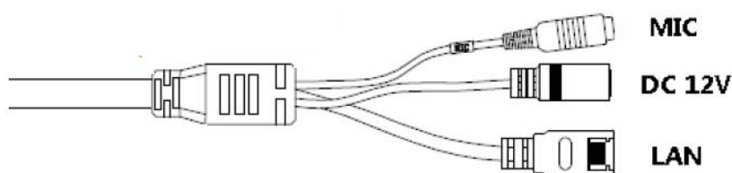
Рис.2.1. Разъемы LTV-ICDMx-E6231L-F
